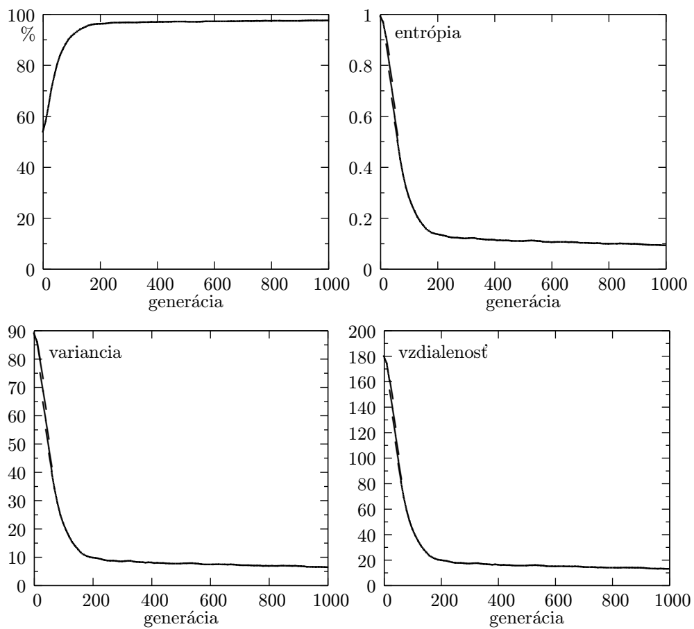
Obr. 10.1: Ukážka konverencie meranej ako percento (vľavo hore), entropia (vpravo hore), variancia (vľavo dole) a vzdialenosť (vpravo dole).
