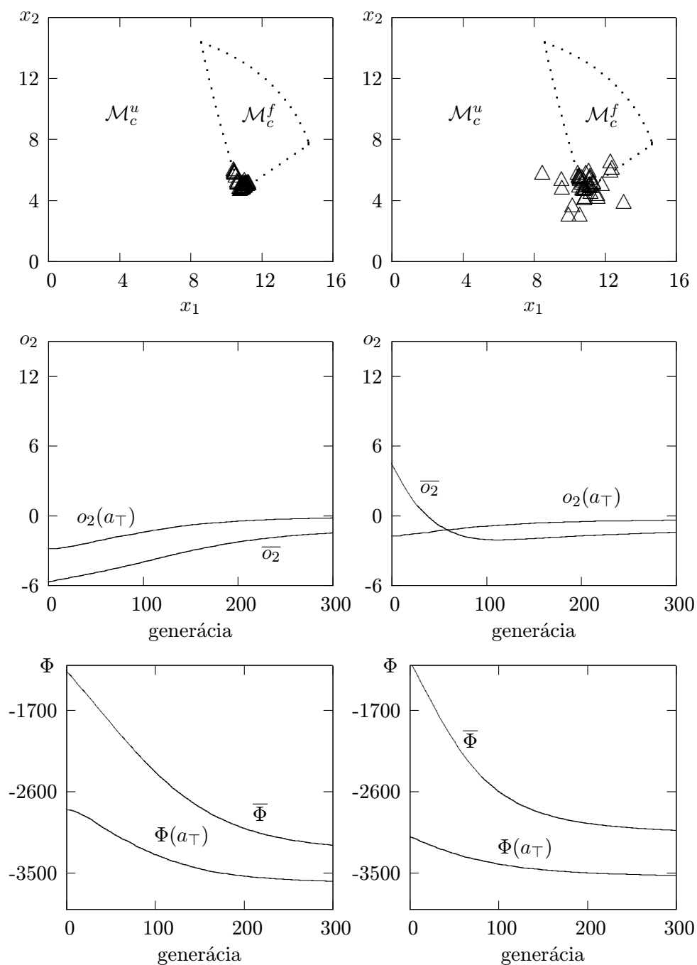
Obr. 4.10: Výsledky pre metódu špeciálneho dekodéra (vľavo) a opravnej procedúry (vpravo).
